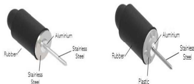
Rivestop typ SS med ändbricka av rostfritt stål.
