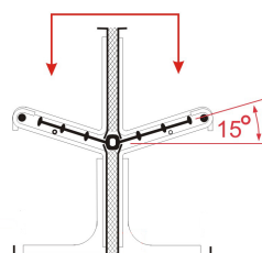
Montera toppdelen på plats över fogbandet
