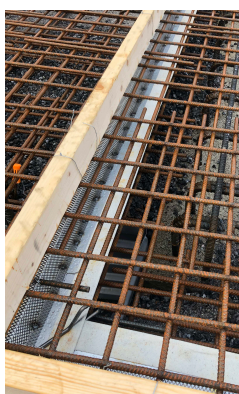
Avstängare 7A, FB monterad för gjutning
