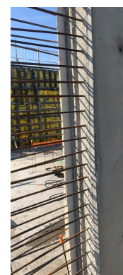
Väggevstängare 7F, FB med betongdistans efter gjutning
