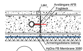
6A Avstängare bottenplatta
