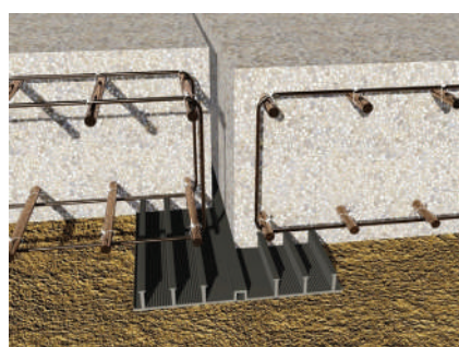
Typ DA/AD, utvändig rörelsefog
