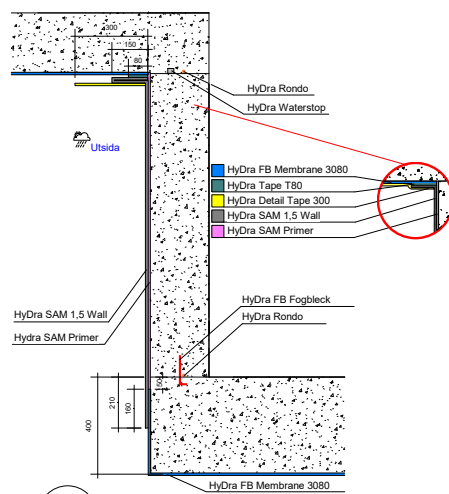
1A Hissgrop eftermonterad
