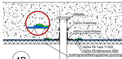
4B Påltopp detalj
