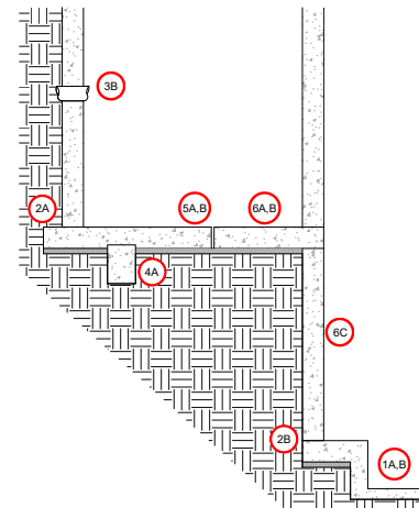
2 Detalj platta/vägg
