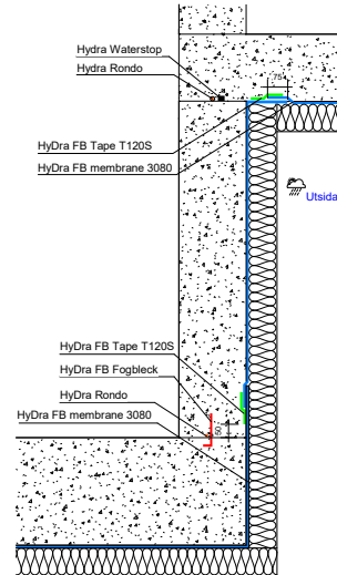
1B Hissgrop förmonterat
