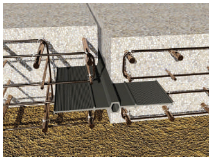
Typ D, invändig rörelsefog
