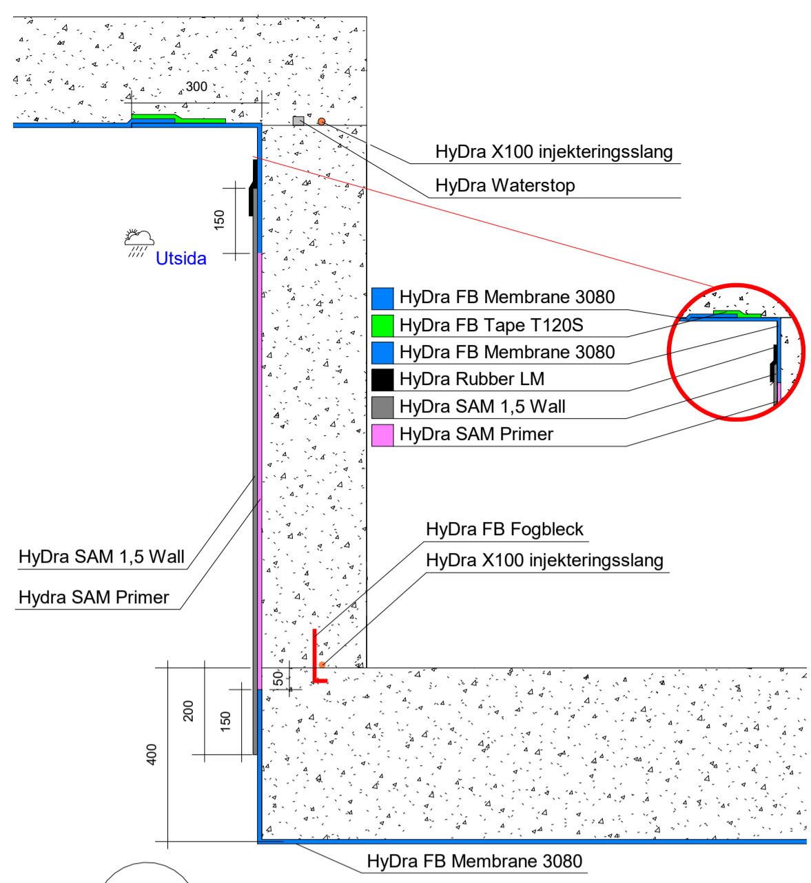
1A Hissgrop eftermonterad
