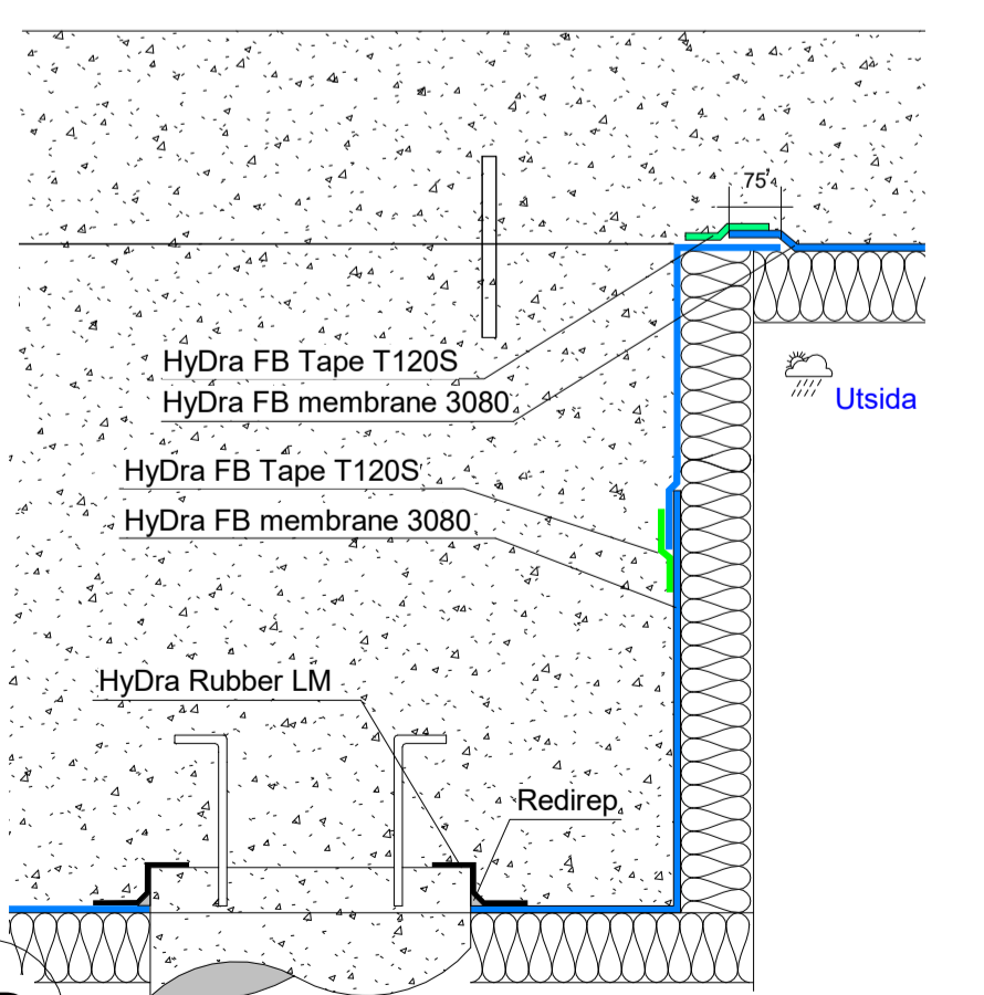
7B Fundament bottenplatta förmonterat
