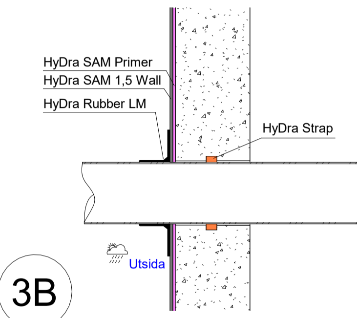
3A Rör genomföringar platta
