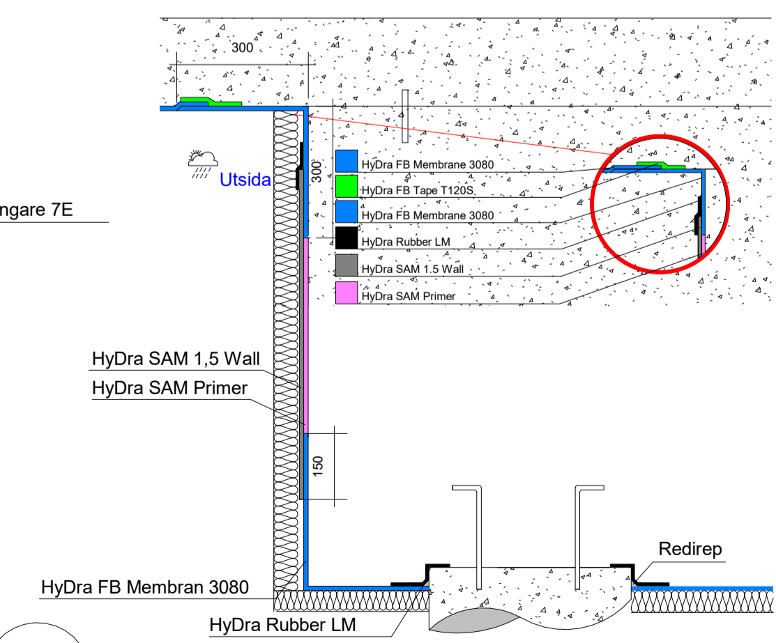
7A Fundament bottenplatta eftermonterad
