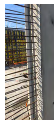
Väggavstängare Nr.7 HyDra FB med betongdistans efter gjutning
