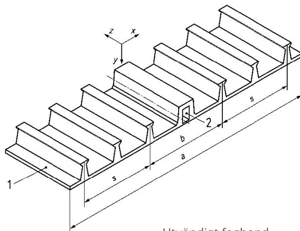
Utvändigt fogband
