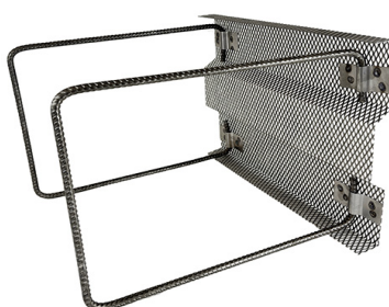
Avstängare Nr.2 med sluten montagebygel och förtagning
